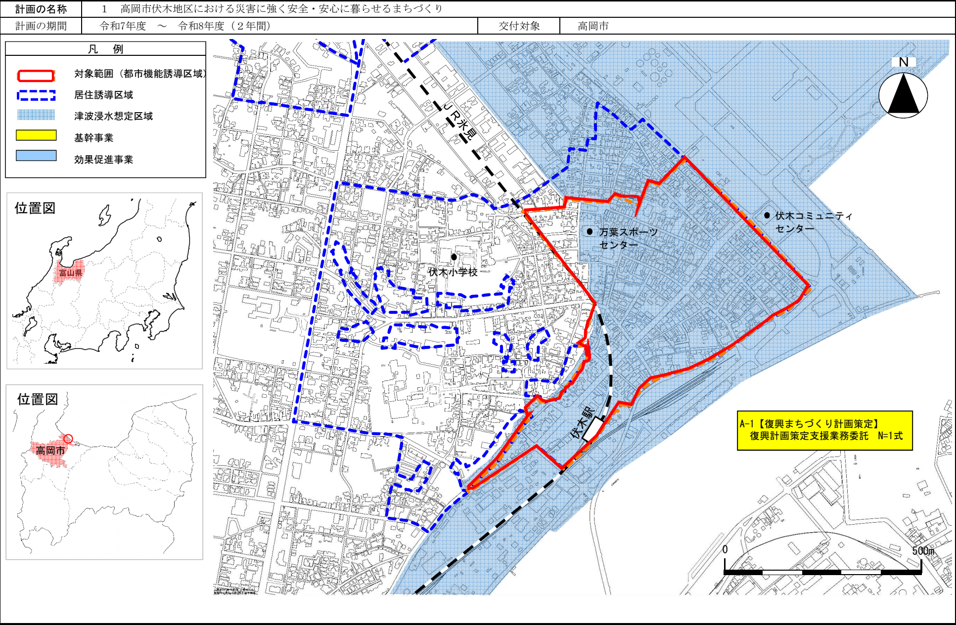
(参考図面)
