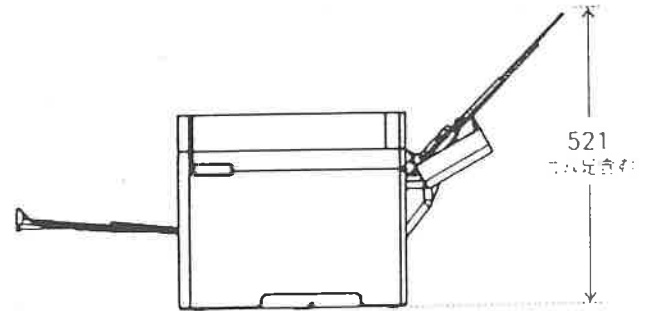
PX-M6011F 使用時 側面図
