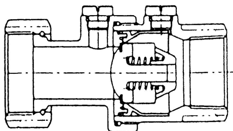
図-3.10.4.3 単式逆止弁
