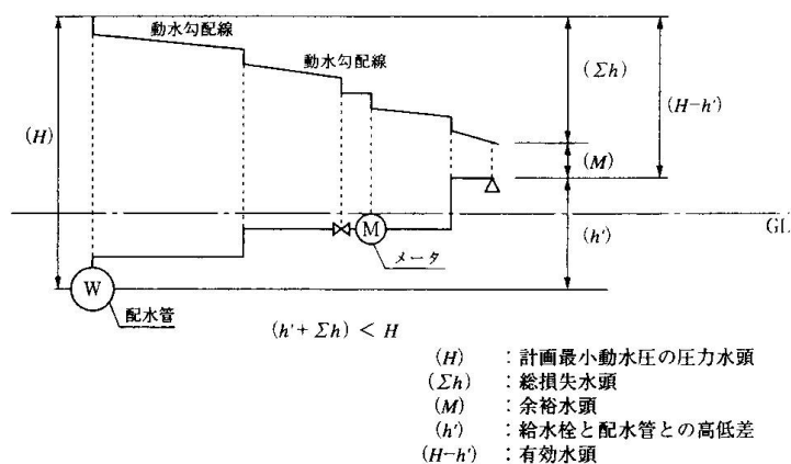
図-2.4.1 動水勾配線図
