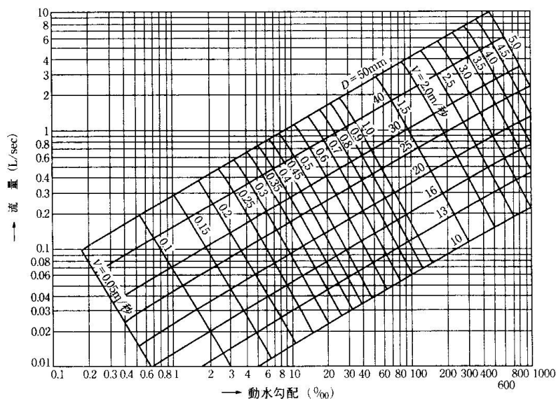
図-2.4.3 ウエストン公式による給水管の流量図
