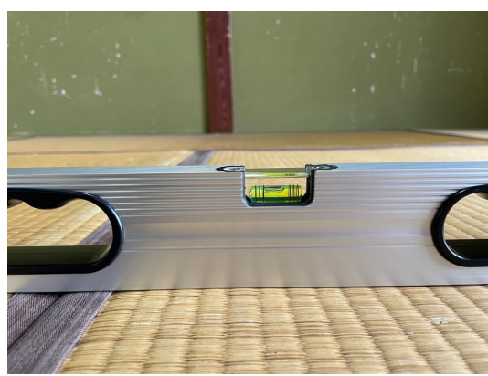
近景：気泡が2メリ目にかかる(約 1/100)
