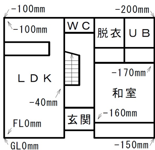
傾斜測定図（業者が作成したものに限る）
