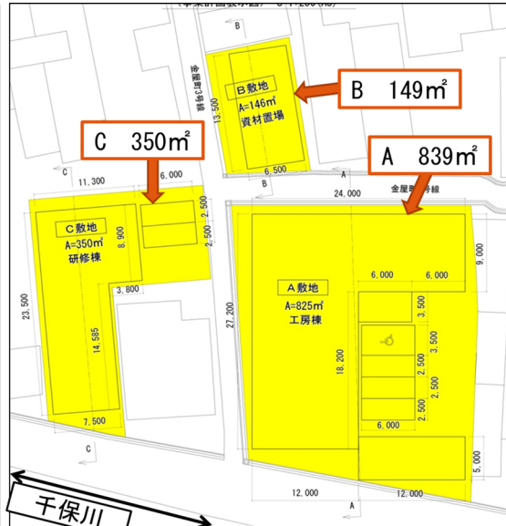
建物配置計画図
