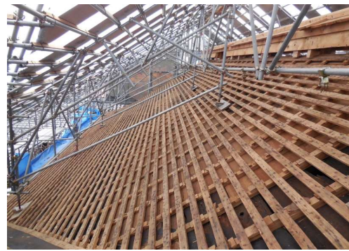
【大茶堂・高廊下】既存こけら板撤去 ②
