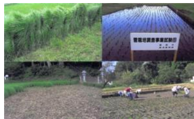
菅栽培調査
