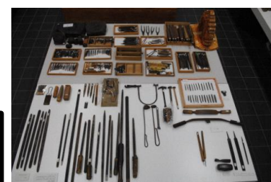
高岡鋳物の製作用具及び製品
