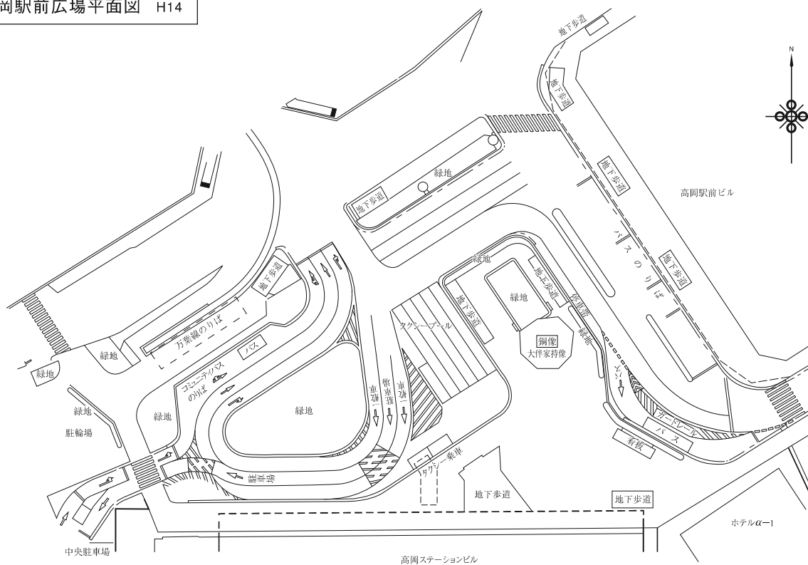
高岡駅前広場平面図 H14
