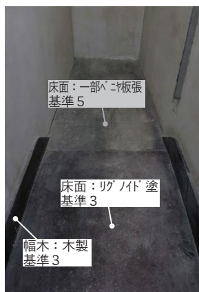
床面
