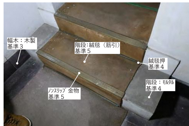
床面（階段）
