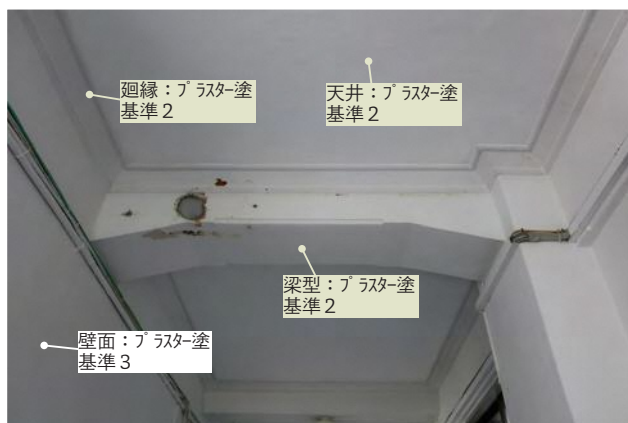
天井面
