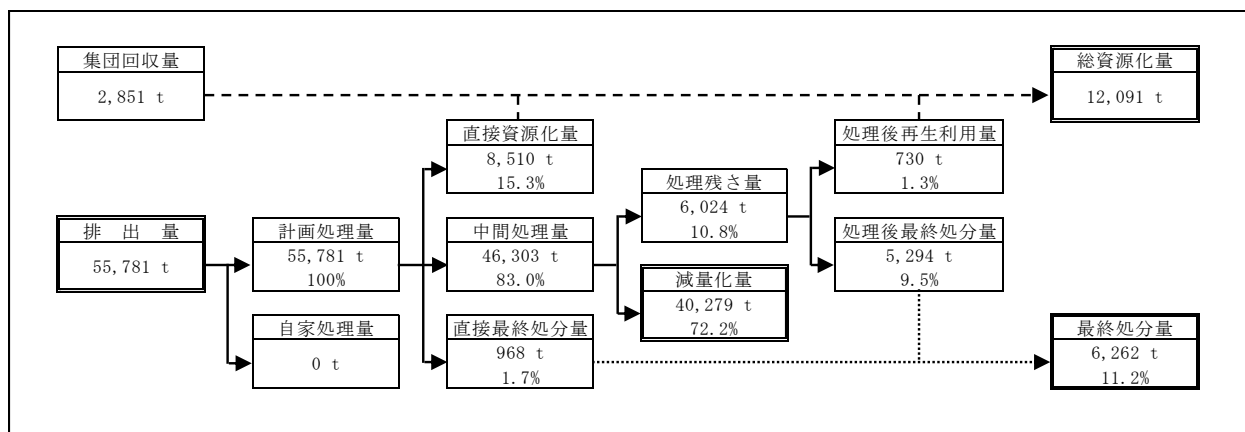
図3-8-1 2021（令和3）年度一般廃棄物の処理状況フロー
