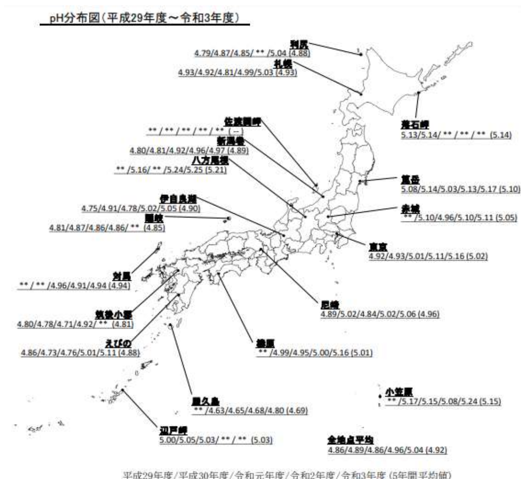
□ 全国の降水の pH 分布図
