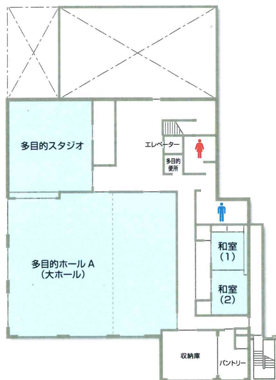
2階 平面図
